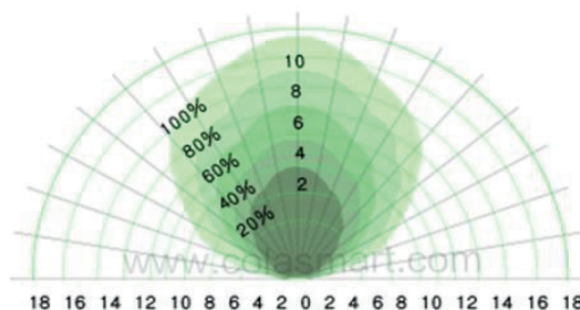
Plafond montage Hoogte installatie 3 Meter
